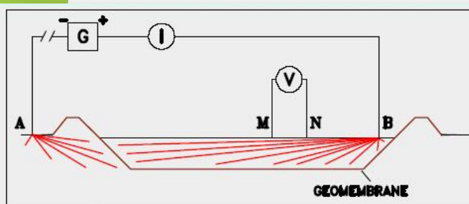
Figura 1 Distribuzione del campo elettrico in condizioni di buon isolamento A-B Elettrodi di corrente M-N Elettrodi di potenziale
