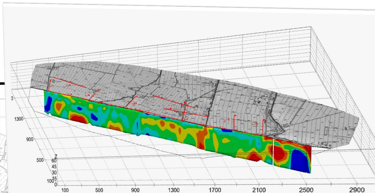
Sezione Verticale
