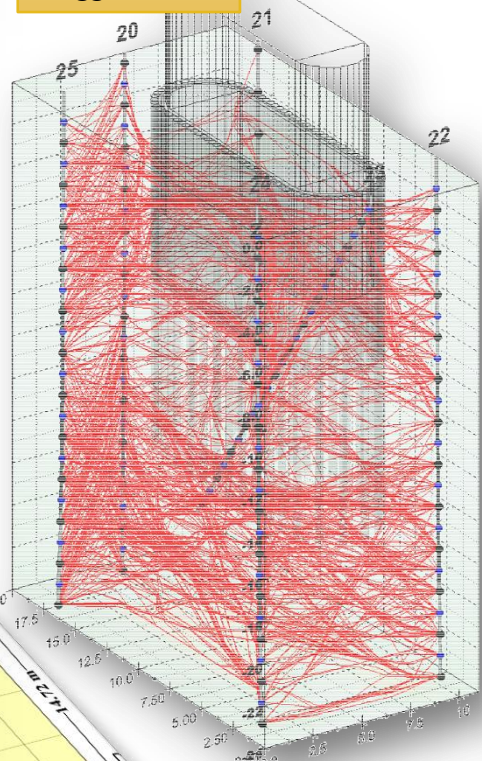
Percorso Raggi Sismici
