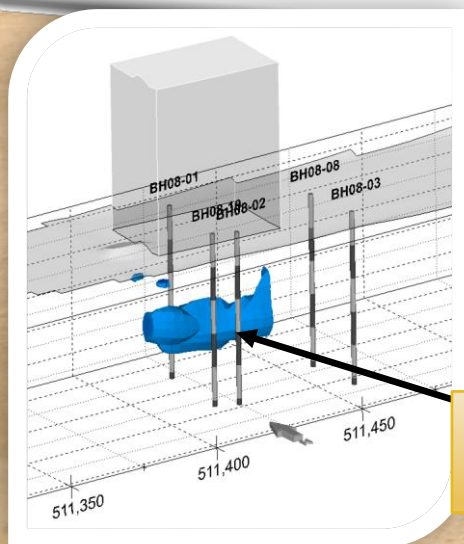
Sovrapposizione Rilievo Tomografico Elettrico Stralcio Isovolum < 0.2 \text{ ohm.m}
