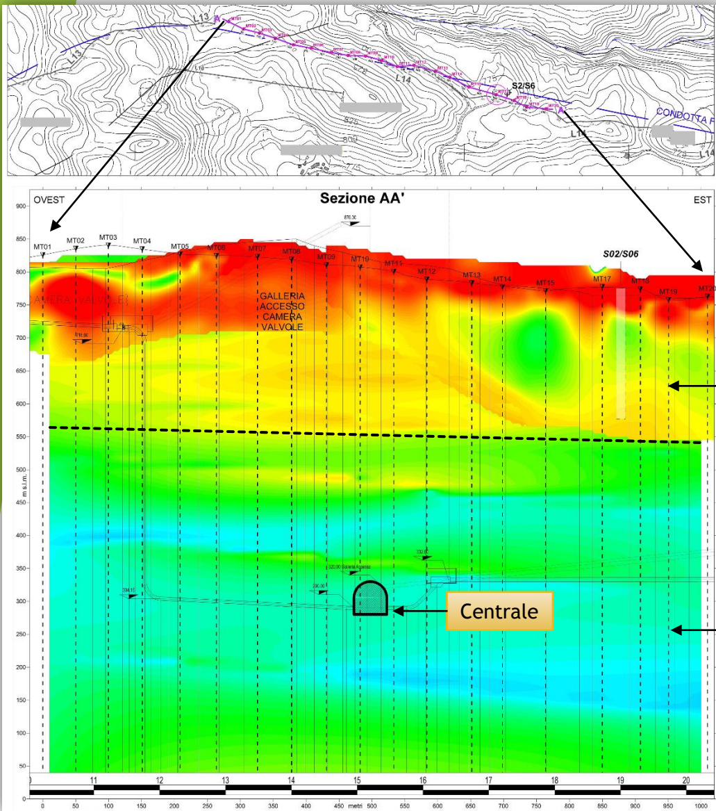
Tomografia Elettrica
